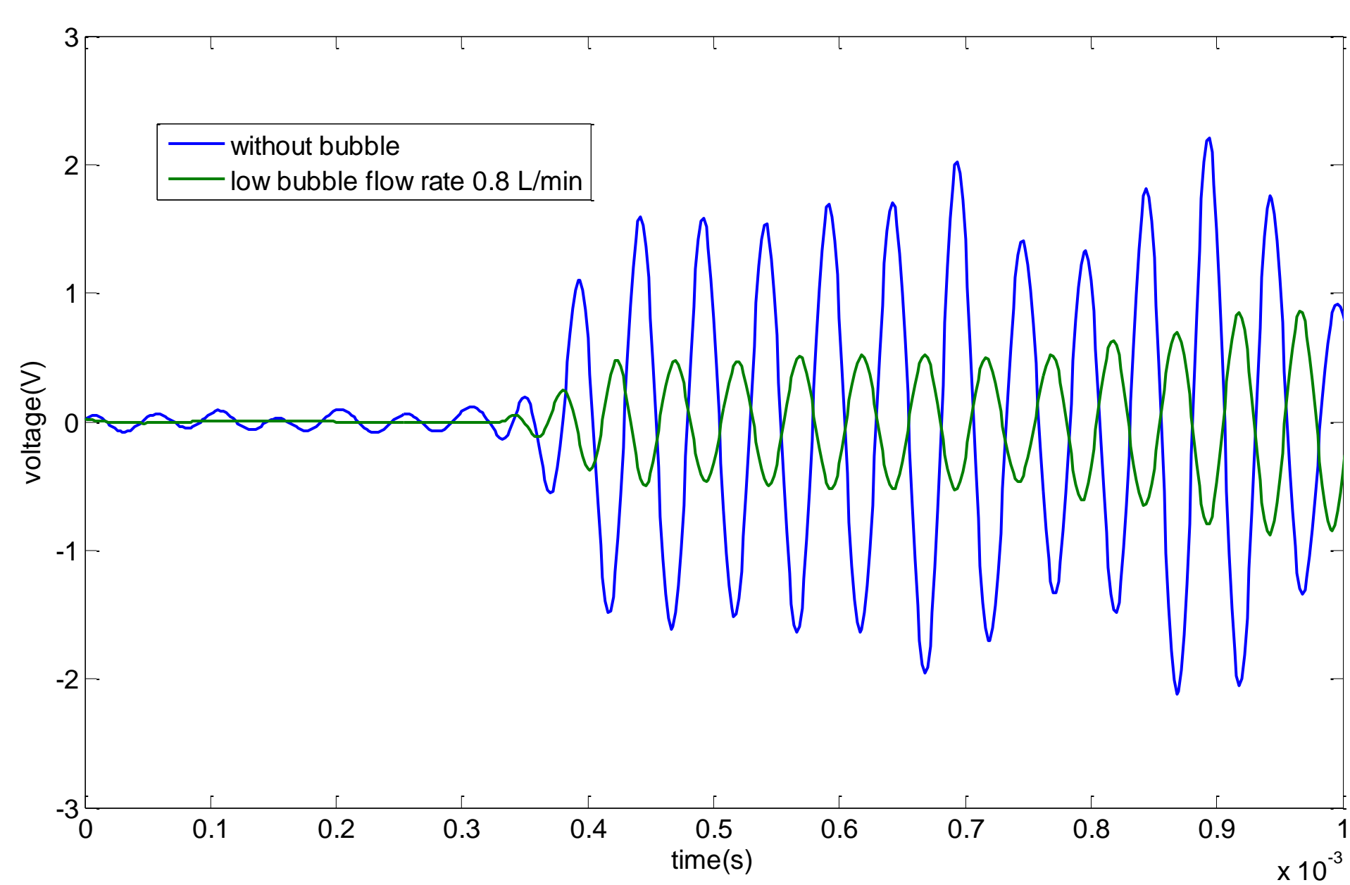
圖2 20 kHz 聲波通過低流量氣泡幕之消音現象
