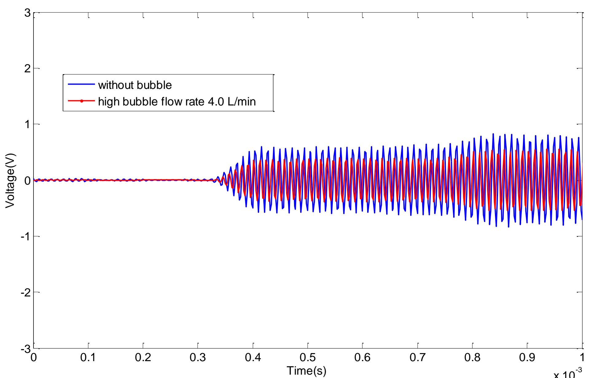
圖3 90 kHz 聲波通過高流量氣泡幕之消音現象
