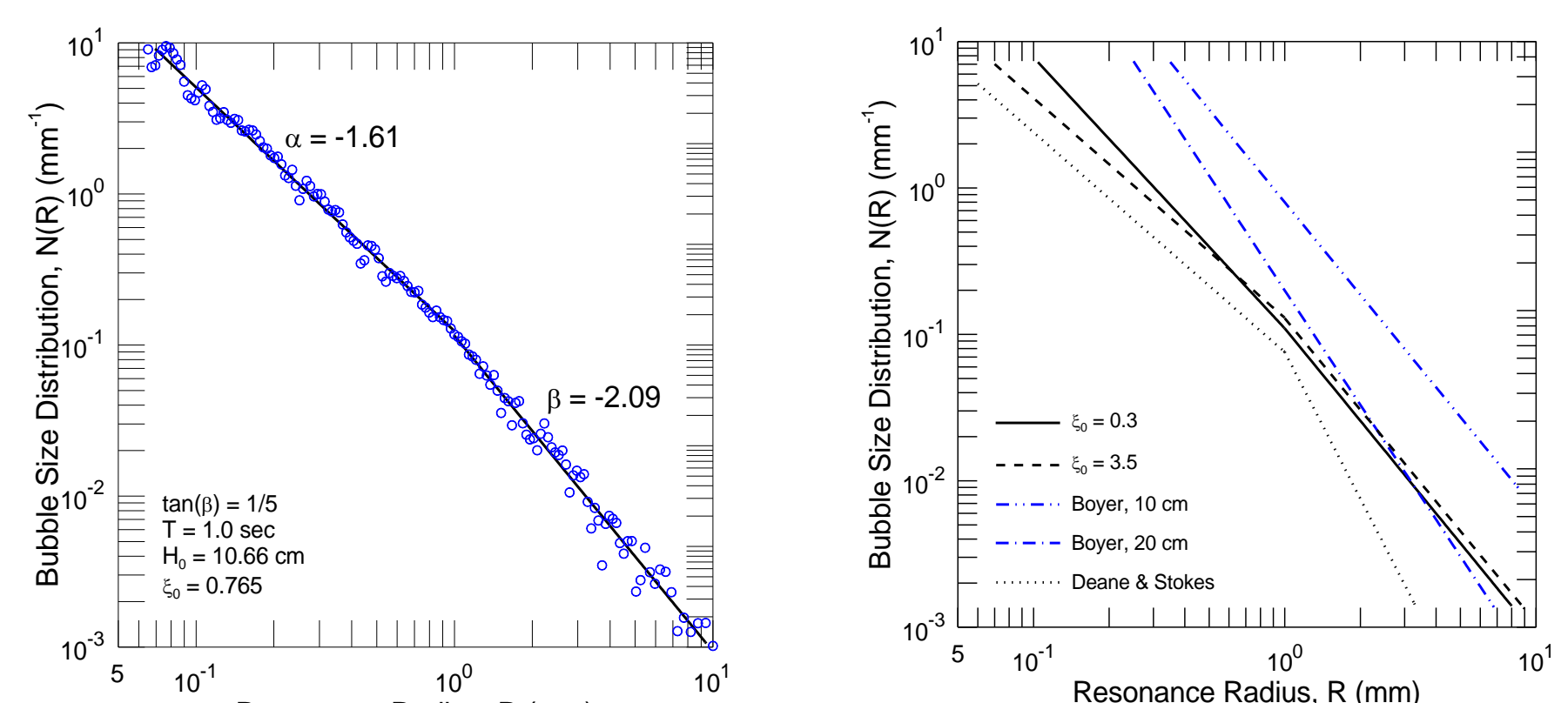
圖8 近岸不同型態碎波捲入氣泡大小特性
