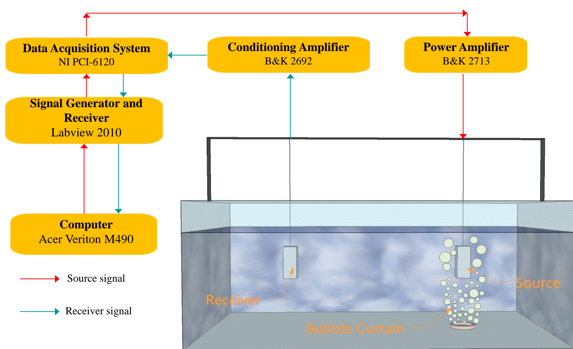
圖1 聲波通過環形氣泡幕衰減特性實驗示意圖
