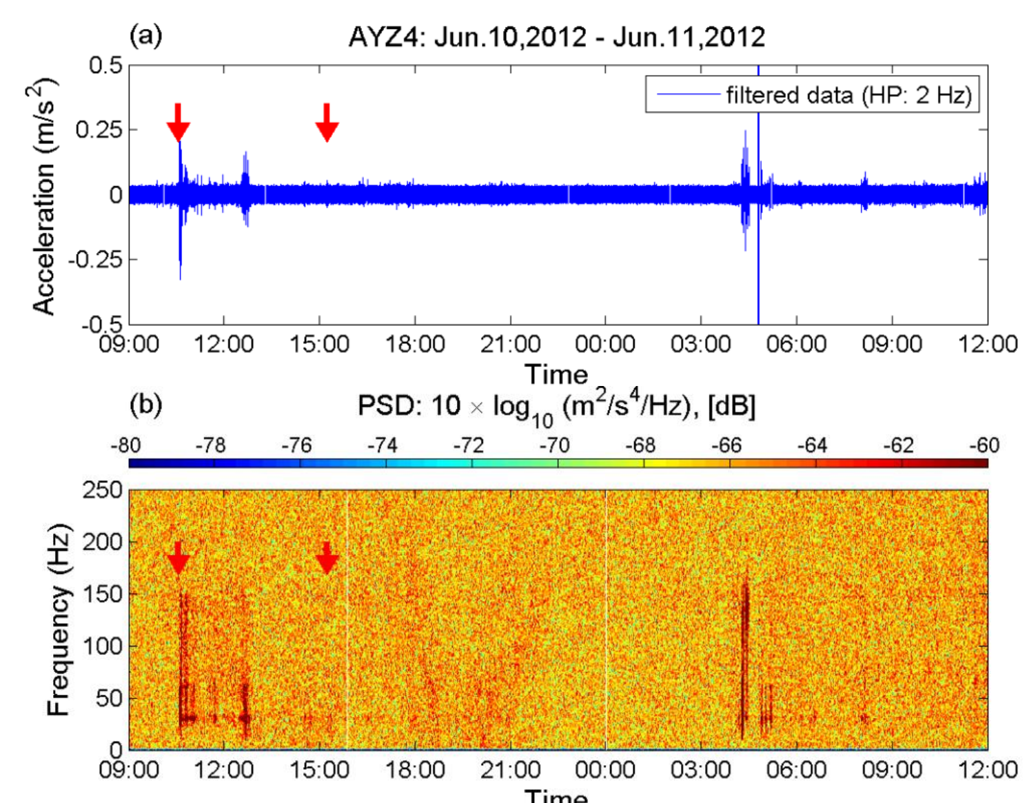
圖5 光纖系統測得土石流地表震動訊號與時頻譜分析結果
