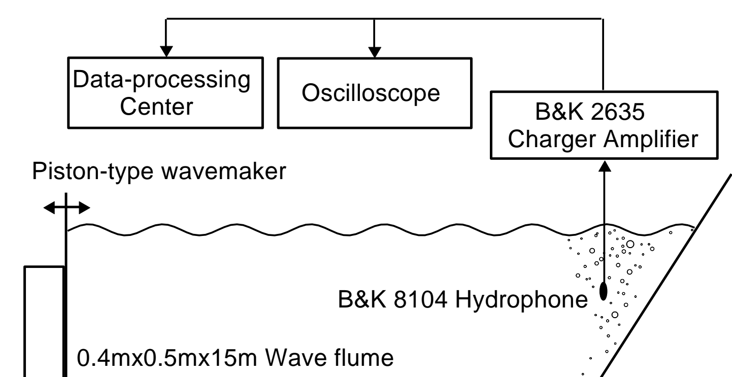
圖6 近岸碎波氣泡特性實驗示意圖
