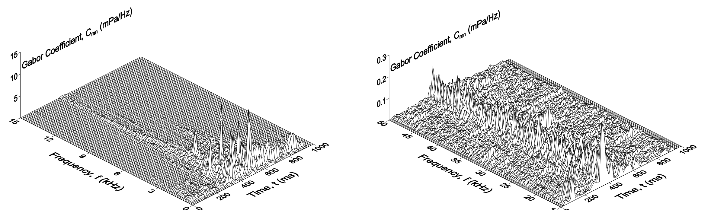
圖7 碎波時所測得水中噪音之時域訊號轉換成時間-頻率域訊號
