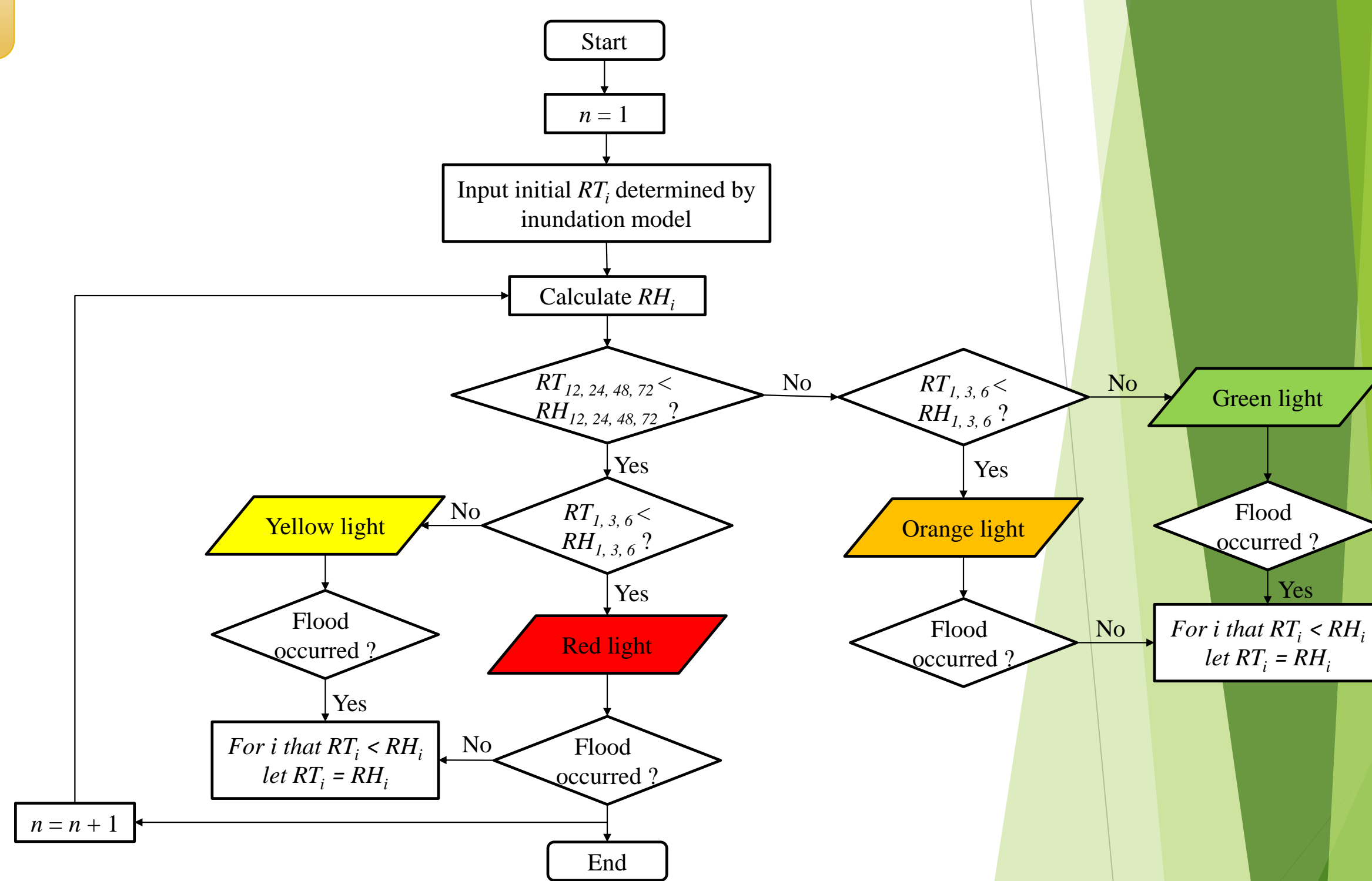
淹水預警燈號判定流程圖
